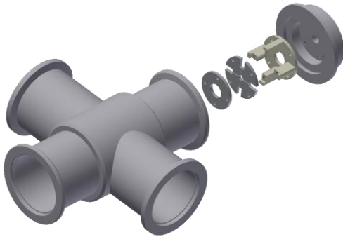
Abb.: Detailansicht der Baugruppe für das Blendensystem.
