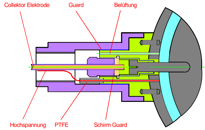
Ansicht "A"
