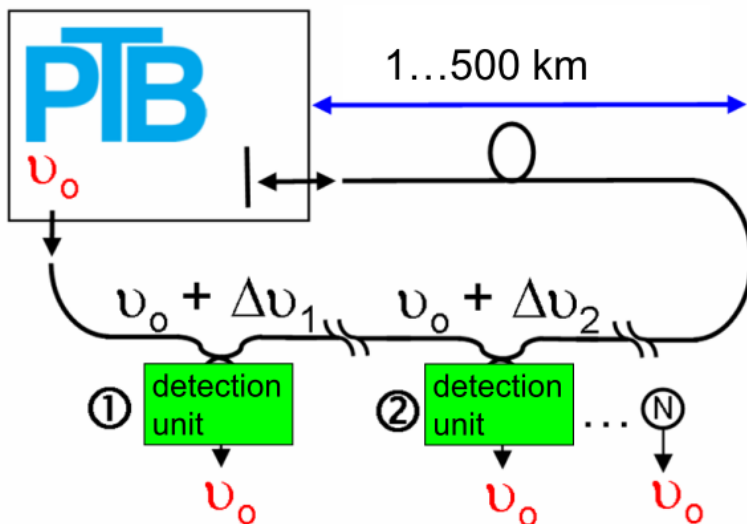
Abbildung 3: Fasergeführte Verteilung ultrapräziser Frequenzsignale an viele Empfänger, indem viele Empfänger auf die gleiche Glasfaserstrecke zugreifen. Jeder Empfänger kann durch eine spezielle Empfangsvorrichtung (detection unit) trotz Übertragungsstörungen das ursprüngliche hochpräzise Frequenzsignal regenerieren [Gro10]. (adaptiert aus – Smandek/Grosche http://www.ptb.de/s/c/tVmXF_Cx/patentDB_Dokumente/A276.pdf )
