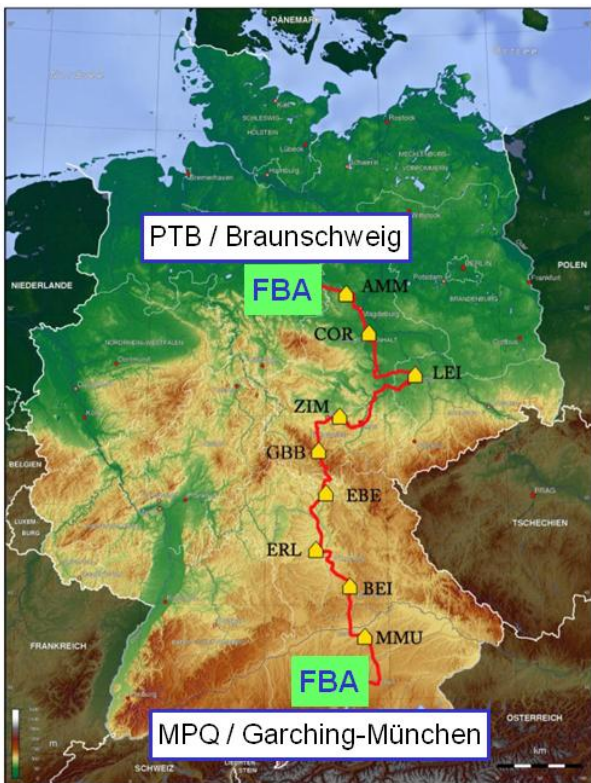
Abbildung 2: Eingebaute Verstärker in der Glasfaserverbindung zur Frequenzübertragung zwischen der PTB, Braunschweig und dem Max-Planck Institut für Quantenoptik in Garching nahe München: EDFAs (gelb) in Containerstandorten entlang der Strecke und FBA (grün) an den Endpunkten. Die gesamte Faserstrecke von 920 km Länge bildet den langen Arm eines Interferometers wie er in Abb. 1 gezeigt ist. [Quelle: adaptiert aus - Katharina Predehl, "A 920 km Optical Fiber Link for Frequency Metrology at the 19th Decimal Place, Doktorarbeit an der LMU München", 2012.]
