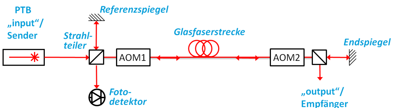
Abbildung 1: Prinzipskizze des Aufbaus für die Frequenzübertragung per Glasfaser, schematisch als Michelson-Interferometer. AOM1 und AOM2 sind akusto-optische Modulatoren, die eine kontrollierbare Frequenzverschiebung bewirken. Zusammen mit der Glasfaserstrecke bilden sie den langen Interferometer-Arm, dessen Phasenexkursionen relativ zum Referenzarm (Strahlteiler/Referenzspiegel) aus dem Schwebungssignal am Fotodetektor bestimmt werden. Eine spezielle Regelektronik (nicht gezeigt) kann den AOM1 so steuern, dass die Lichtphase im langen Interferometerarm nicht fluktuiert. So liegt am Endspiegel und damit auch am Empfänger Ausgang eine konstante und bekannte Frequenz vor: die Glasfaserstrecke ist „stabilisiert“.
