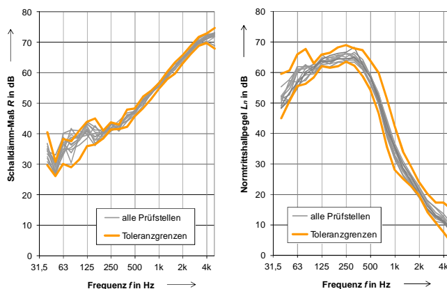
Bild 3: Messergebnisse der Prüfstellen für Luft- und Trittschall
