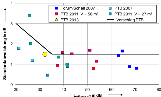
Bild 8: Vorschlag der PTB für die Unsicherheiten des Normschalldruckpegels haustechnischer Anlagen und Ergebnisse der vorliegenden Ringversuche
