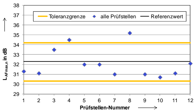
Bild 6: Ergebnisse der Prüfstellen
