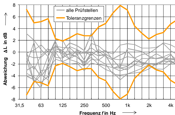
Bild 5: Abweichungen vom Referenzwert, Normtrittschallpegel
