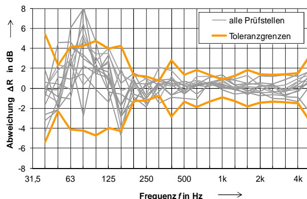
Bild 4: Abweichungen vom Referenzwert, Luftschalldämmmaß
