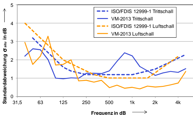
Bild 7: Standardabweichungen der Vergleichsmessungen im Vergleich mit den vorgeschlagenen Unsicherheiten der ISO/FDIS 12999-1 für Luft- und Trittschall
