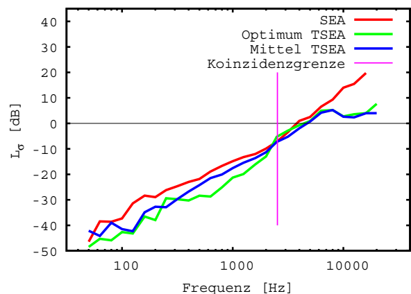
Abbildung 4: Ins Abstrahlmaß L_\sigma umgerechneter Kopplungsverlustfaktor \eta_{21} : nach stationärer Methode gemäß [2] (SEA), nach transienter Methode mit beiden Verfahren (Optimum TSEA) und (Mittel TSEA); dazu die Koinzidenzfrequenz und eine Hilfslinie bei 0 dB
