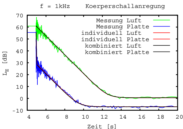
Abbildung 1: Beispiel eines Identifikationsergebnisses; verglichen werden die Messkurven im Luftvolumen (grün) und auf der Platte (blau) mit den Ergebniskurven der individuellen (rot) und der gemeinsamen (schwarz) Identifikation
