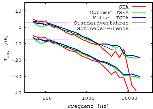
Abbildung 3: Vergleich der Körperschallnachhallzeiten auf der Platte: nach stationärer Methode gemäß [2] (SEA), nach transienter Methode mit beiden Verfahren (Optimum TSEA) und (Mittel TSEA) und nach dem Standardverfahren [6]; dazu die maximal messbare Nachhallzeit (Schröder-Grenze); obere Kurvenschar: \eta_{22} , darunter (-10 dB Versatz): \eta_{2,total}
