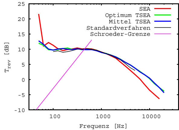
Abbildung 2: Vergleich der Nachhallzeiten im Hallraum: nach stationärer Methode gemäß [2] (SEA), nach transienter Methode mit beiden Verfahren (Optimum TSEA) und (Mittel TSEA) und nach dem Standardverfahren [5]; dazu die maximal messbare Nachhallzeit (Schröder-Grenze)
